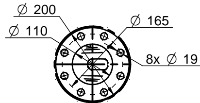
DETALLE B
